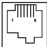
Figure A-4 — Brochage de l'adaptateur MMJ
