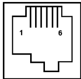
Figure A-4—Pin adattatori MMJ
